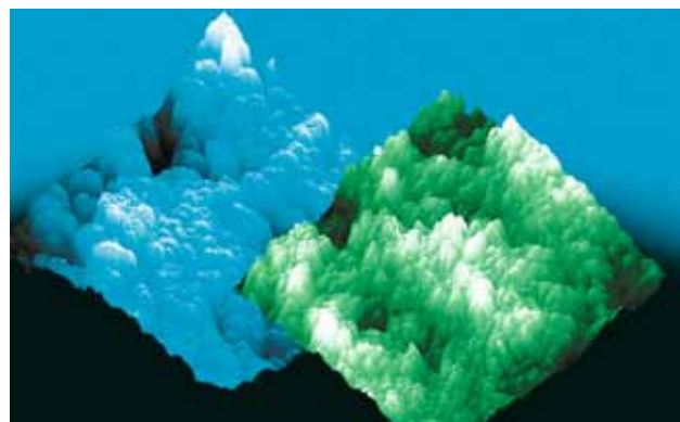
Uno sguardo al microscopio elettronico: a sinistra la superficie di una foglia di loto e a destra la superficie di StoLotusan.
